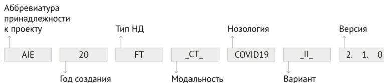
Рисунок 9 – Правила формирования внутреннего идентификатора НД
